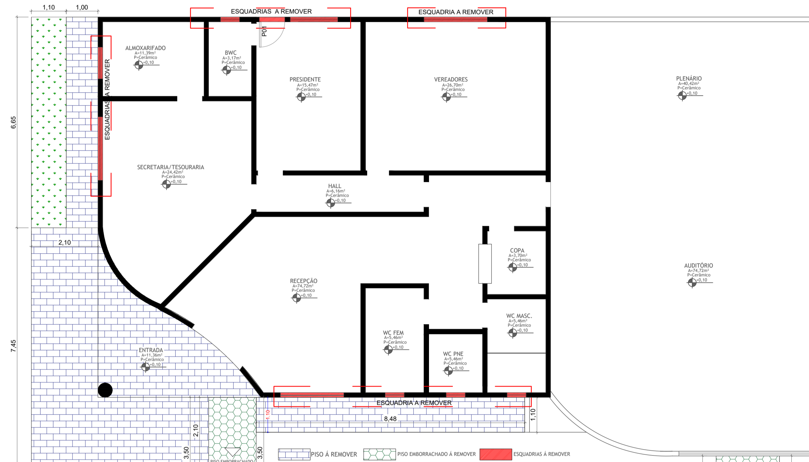
PLANTA BAIXA REFORMA Esc. 1/75
